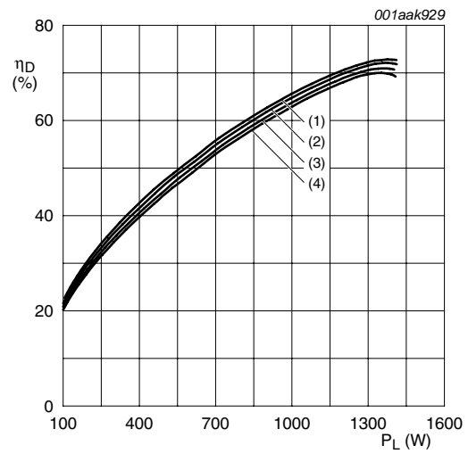
V_{DS} = 50\text{ V} ; f = 225\text{ MHz} ; t_p = 100\text{ }\mu\text{s} ; \delta = 20\% . (1) I_{Dq} = 0\text{ mA} (2) I_{Dq} = 40\text{ mA} (3) I_{Dq} = 80\text{ mA} (4) I_{Dq} = 160\text{ mA}
