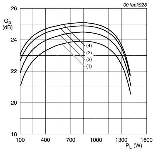
V_{DS} = 50\text{ V} ; f = 225\text{ MHz} ; t_p = 100\text{ }\mu\text{s} ; \delta = 20\% . (1) I_{Dq} = 0\text{ mA} (2) I_{Dq} = 40\text{ mA} (3) I_{Dq} = 80\text{ mA} (4) I_{Dq} = 160\text{ mA}
