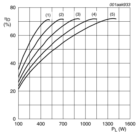
I_{Dq} = 40\text{ mA} ; f = 225\text{ MHz} ; t_p = 100\text{ }\mu\text{s} ; \delta = 20\% . (1) V_{DS} = 30\text{ V} (2) V_{DS} = 35\text{ V} (3) V_{DS} = 40\text{ V} (4) V_{DS} = 45\text{ V} (5) V_{DS} = 50\text{ V}
