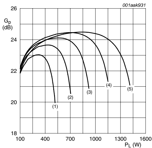
I_{Dq} = 40\text{ mA} ; f = 225\text{ MHz} ; t_p = 100\text{ }\mu\text{s} ; \delta = 20\% . (1) V_{DS} = 30\text{ V} (2) V_{DS} = 35\text{ V} (3) V_{DS} = 40\text{ V} (4) V_{DS} = 45\text{ V} (5) V_{DS} = 50\text{ V}
